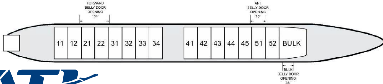
1 CONTAINER PER ROW 15 CENTERLINE ROWS
