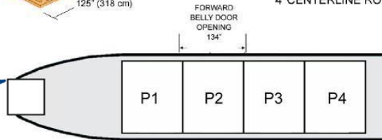
1 CONTAINER PER ROW 4 CENTERLINE ROWS
