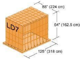
1 CONTAINER PER ROW 4 CENTERLINE ROWS
